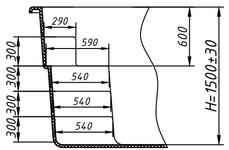
Сечение 2-2
